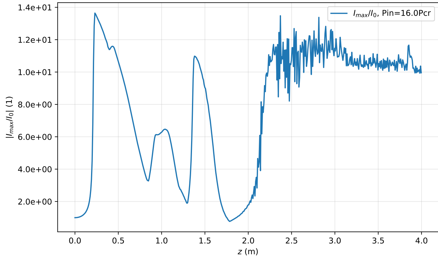
I_{max}(r=0, z)/I_0 , Pin=16.0Pcr
