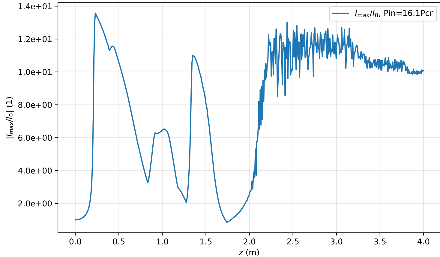
I_{\max}(r=0, z)/I_0 , Pin=16.1Pcr
