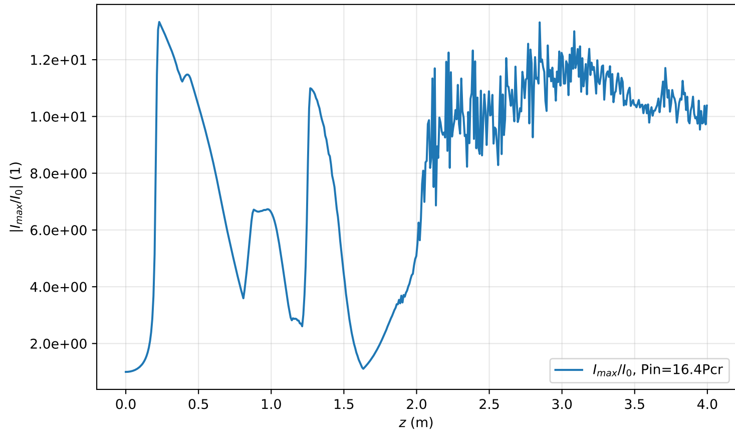
I_{max}(r=0, z)/I_0 , Pin=16.4Pcr
