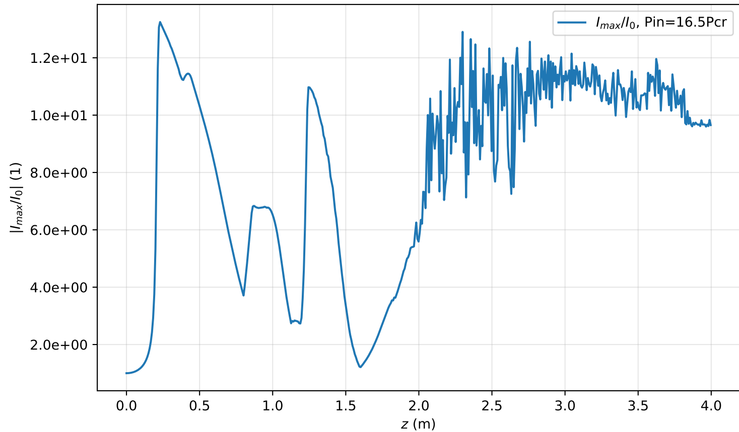
I_{\max}(r=0, z)/I_0 , Pin=16.5Pcr
