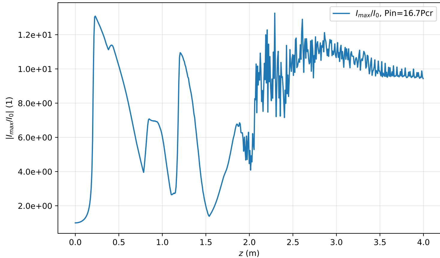
I_{max}(r=0, z)/I_0 , Pin=16.7Pcr
