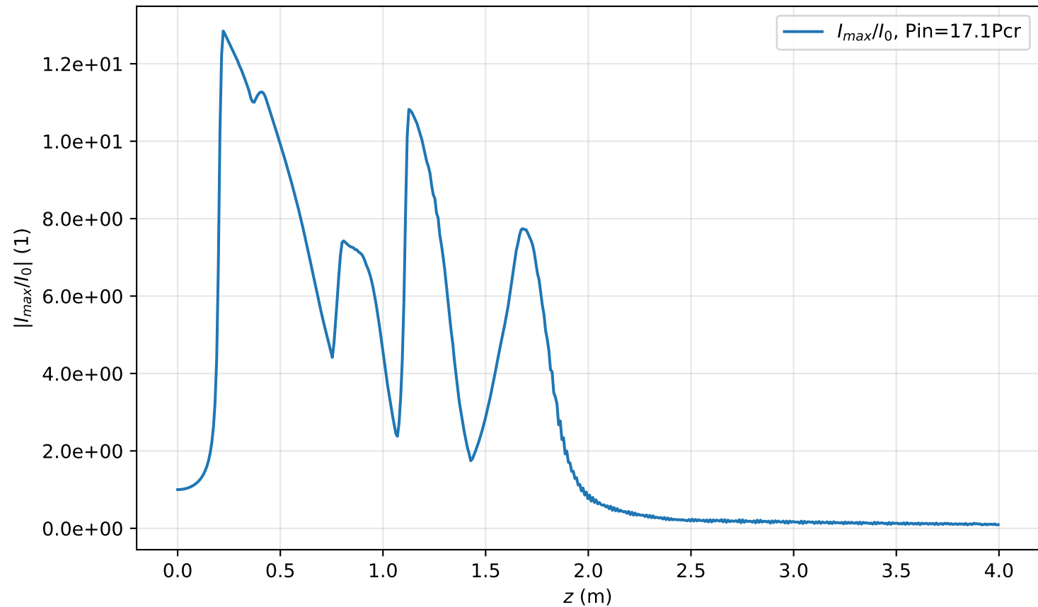
I_{\max}(r=0, z)/I_0 , Pin=17.1Pcr
