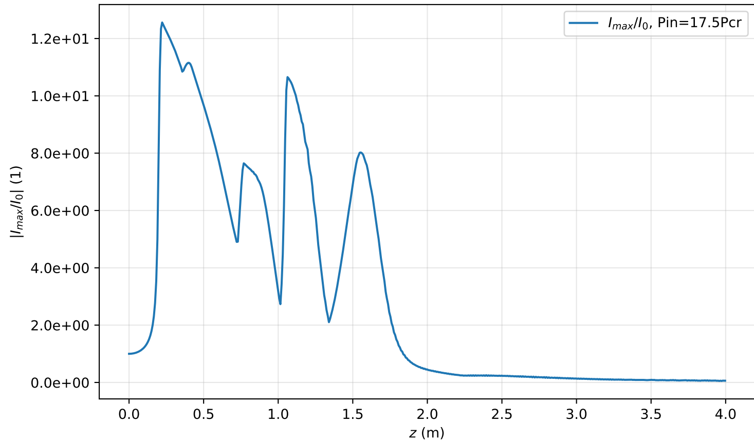
I_{max}(r=0, z)/I_0 , Pin=17.5Pcr
