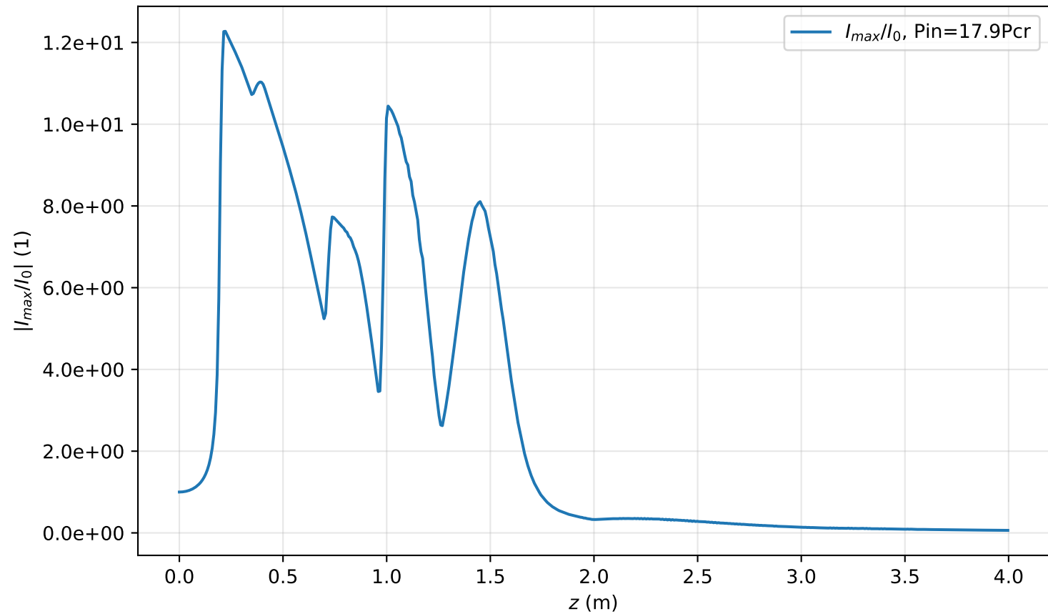
I_{max}(r=0, z)/I_0 , Pin=17.9Pcr
