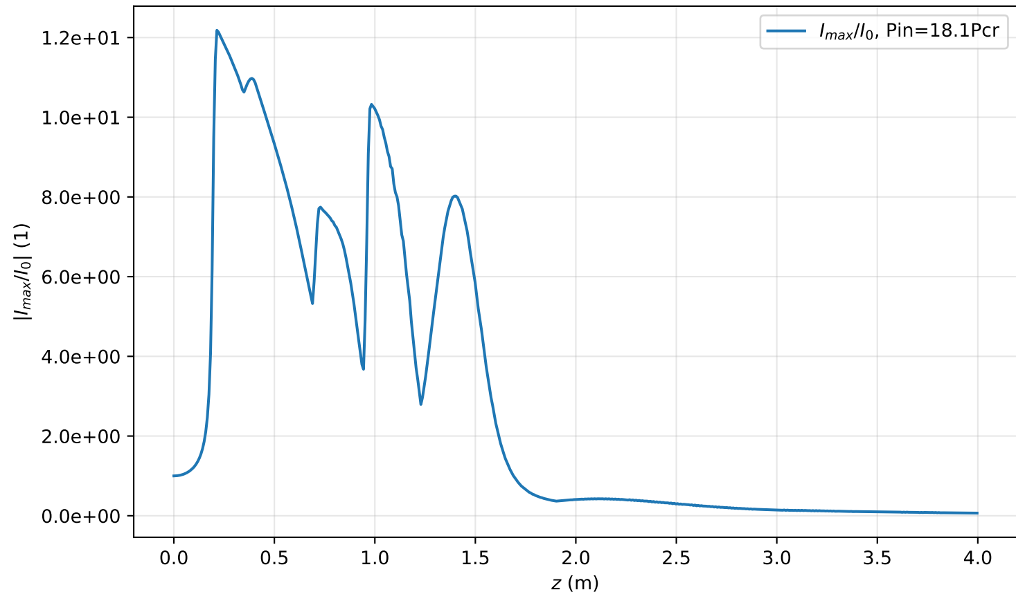
I_{max}(r=0, z)/I_0 , Pin=18.1Pcr
