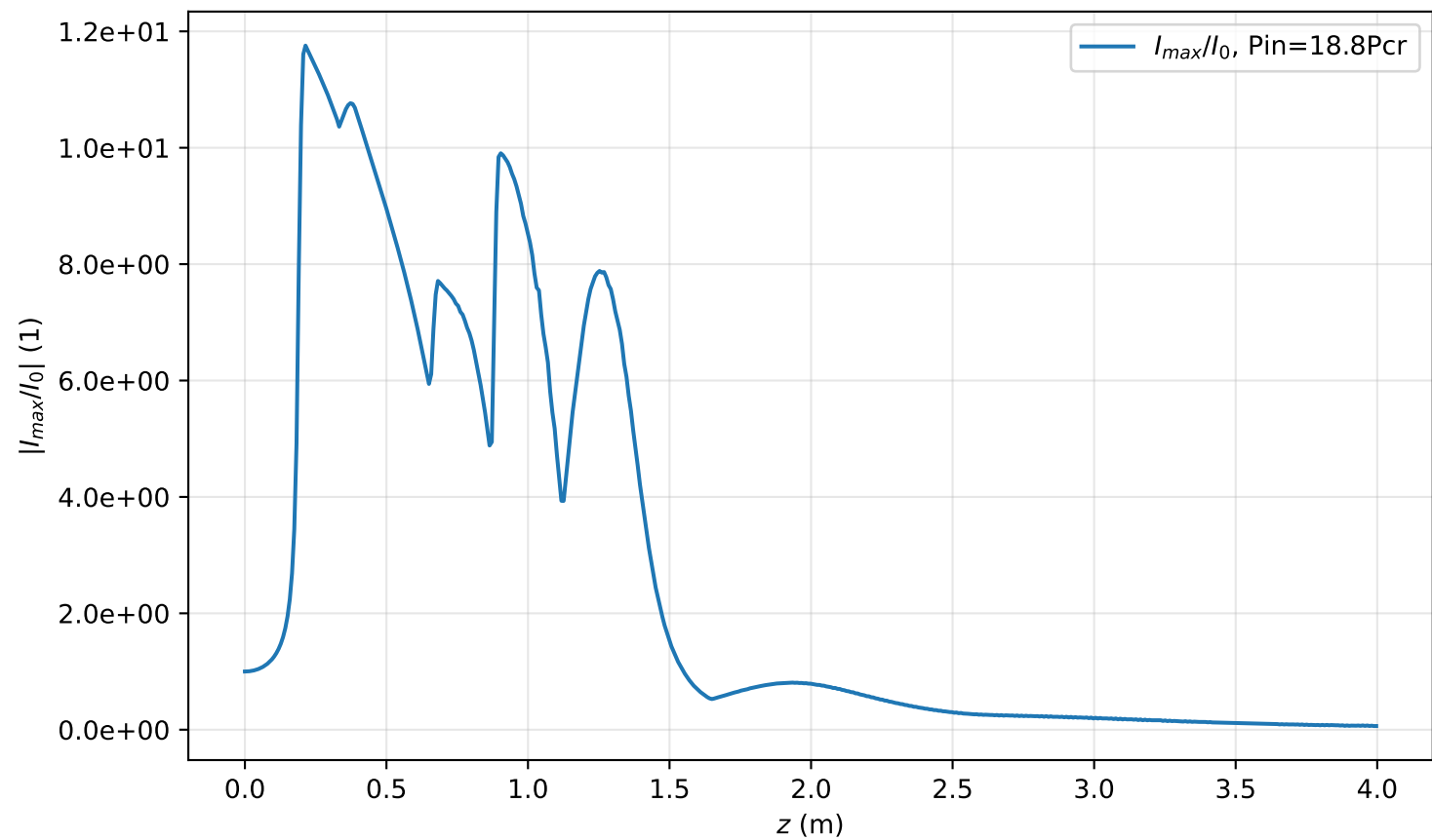
I_{max}(r=0, z)/I_0 , Pin=18.8Pcr
