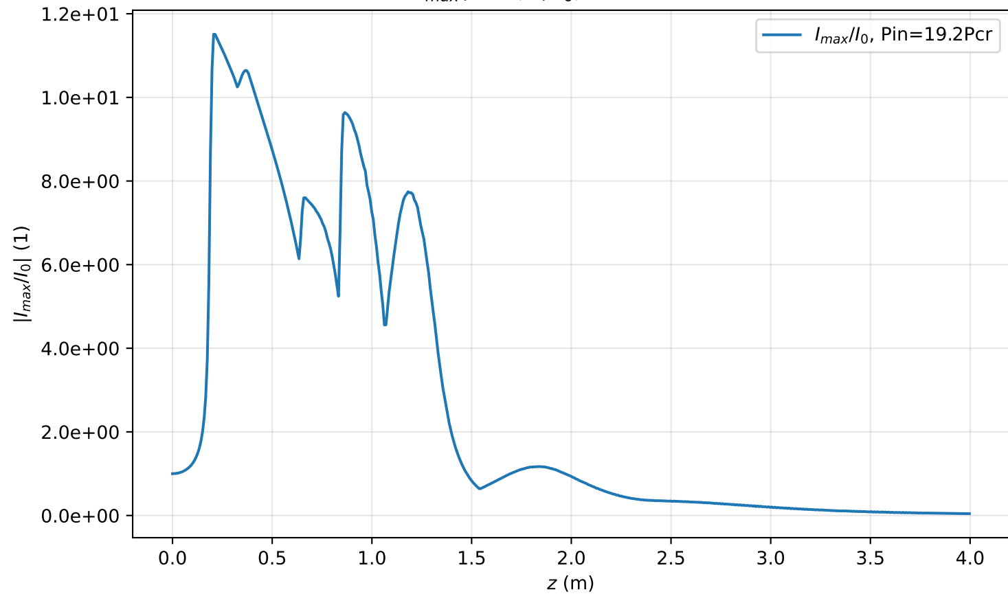
I_{max}(r=0, z)/I_0 , Pin=19.2Pcr
