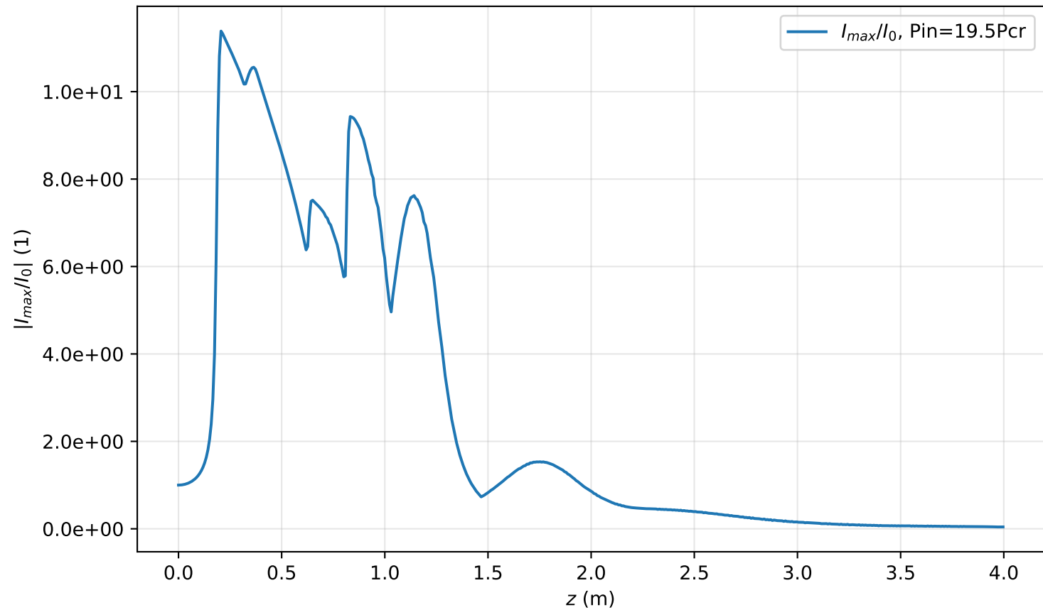
I_{max}(r=0, z)/I_0 , Pin=19.5Pcr
