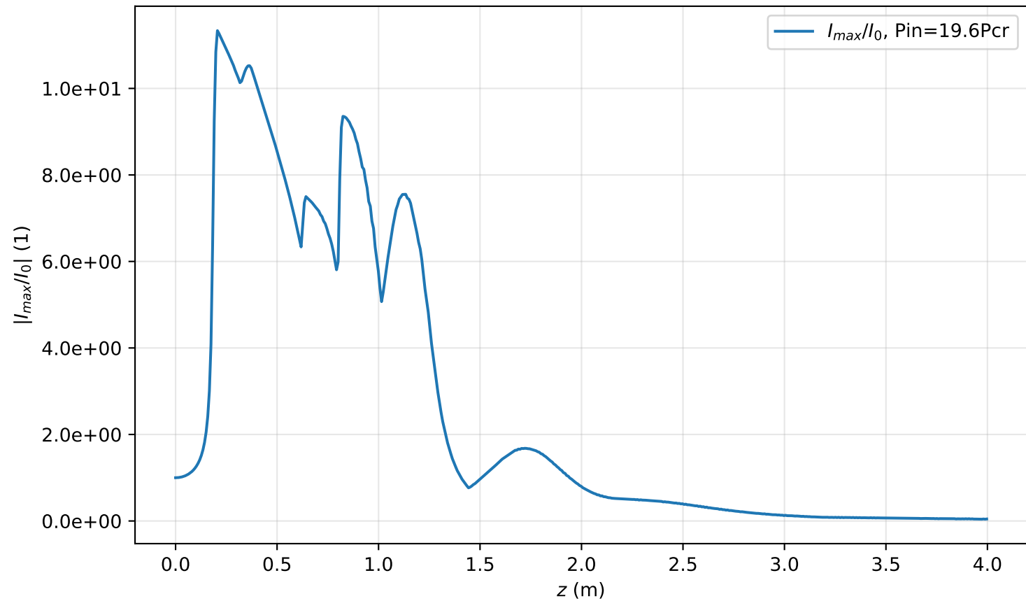
I_{max}(r=0, z)/I_0 , Pin=19.6Pcr
