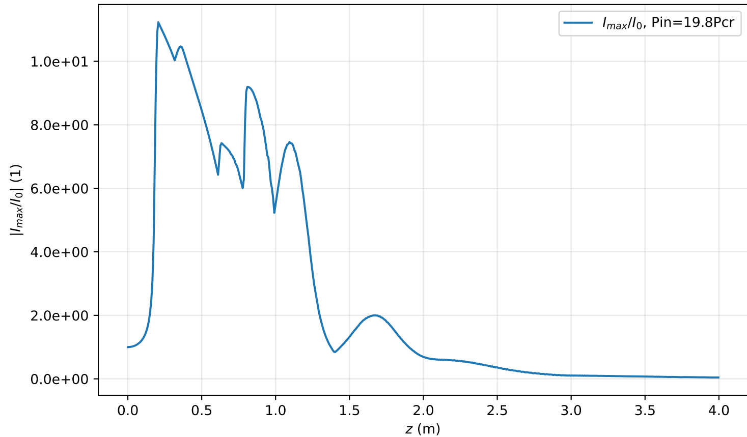
I_{max}(r=0, z)/I_0 , Pin=19.8Pcr
