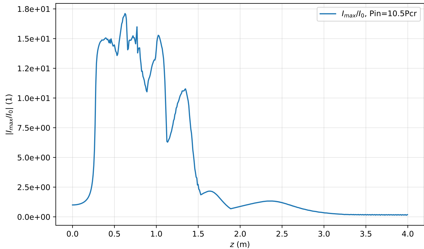
I_{max}(r=0, z)/I_0 , Pin=10.5Pcr
