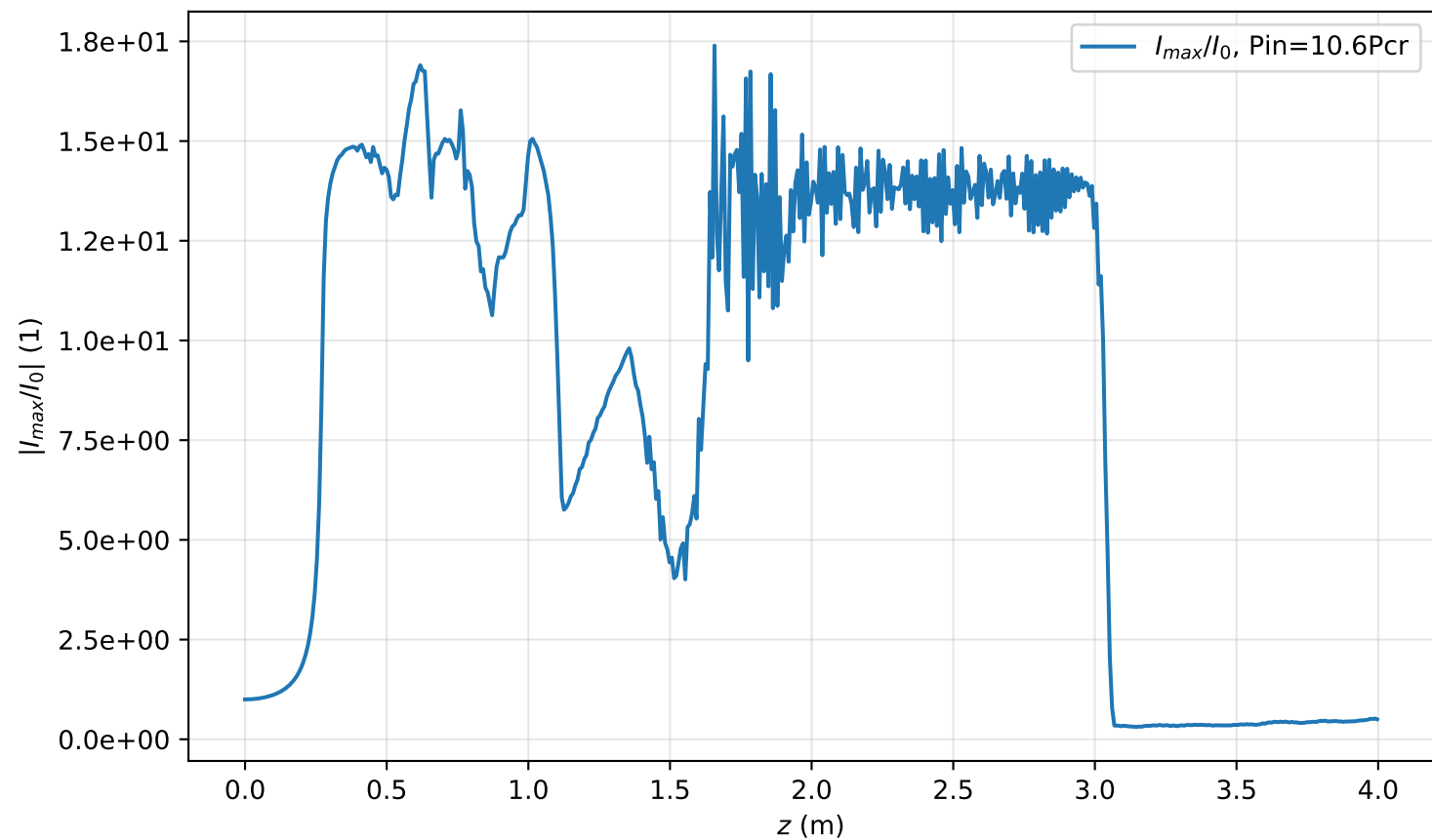
I_{max}(r=0, z)/I_0 , Pin=10.6Pcr
