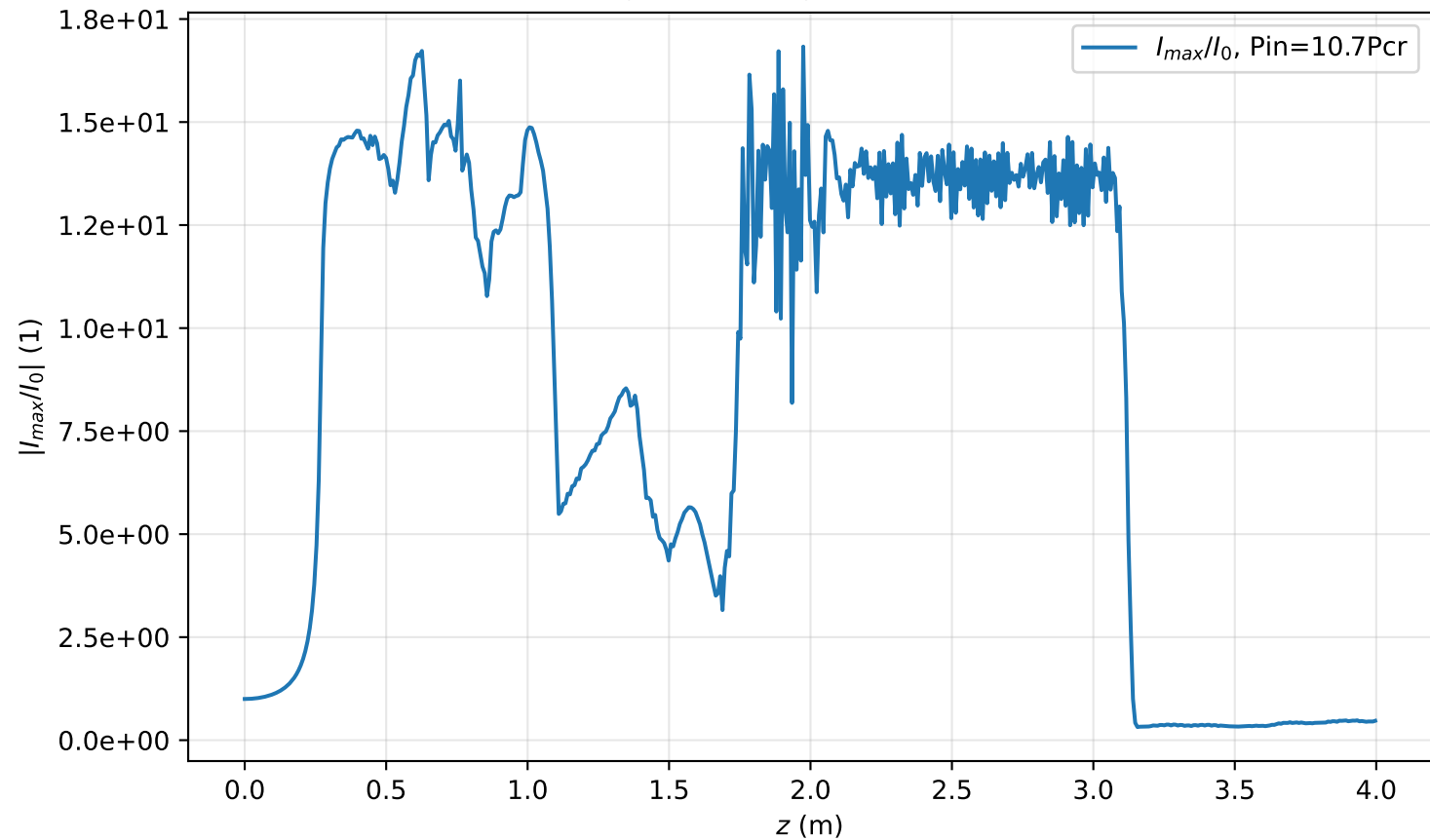
I_{max}(r = 0, z)/I_0 , Pin=10.7Pcr
