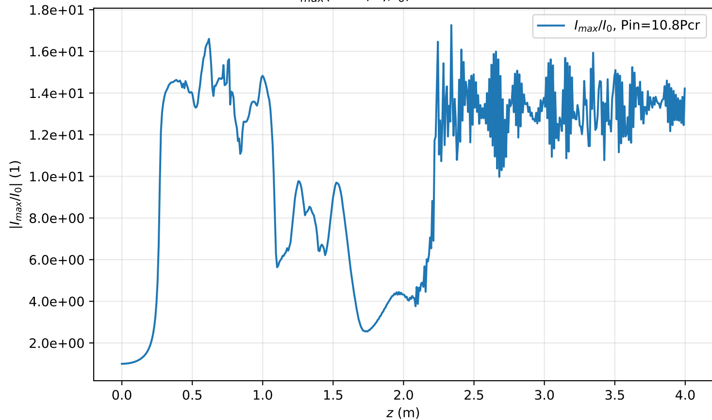
I_{max}(r=0, z)/I_0 , Pin=10.8Pcr
