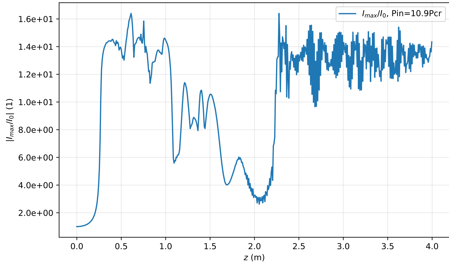
I_{max}(r=0, z)/I_0 , Pin=10.9Pcr
