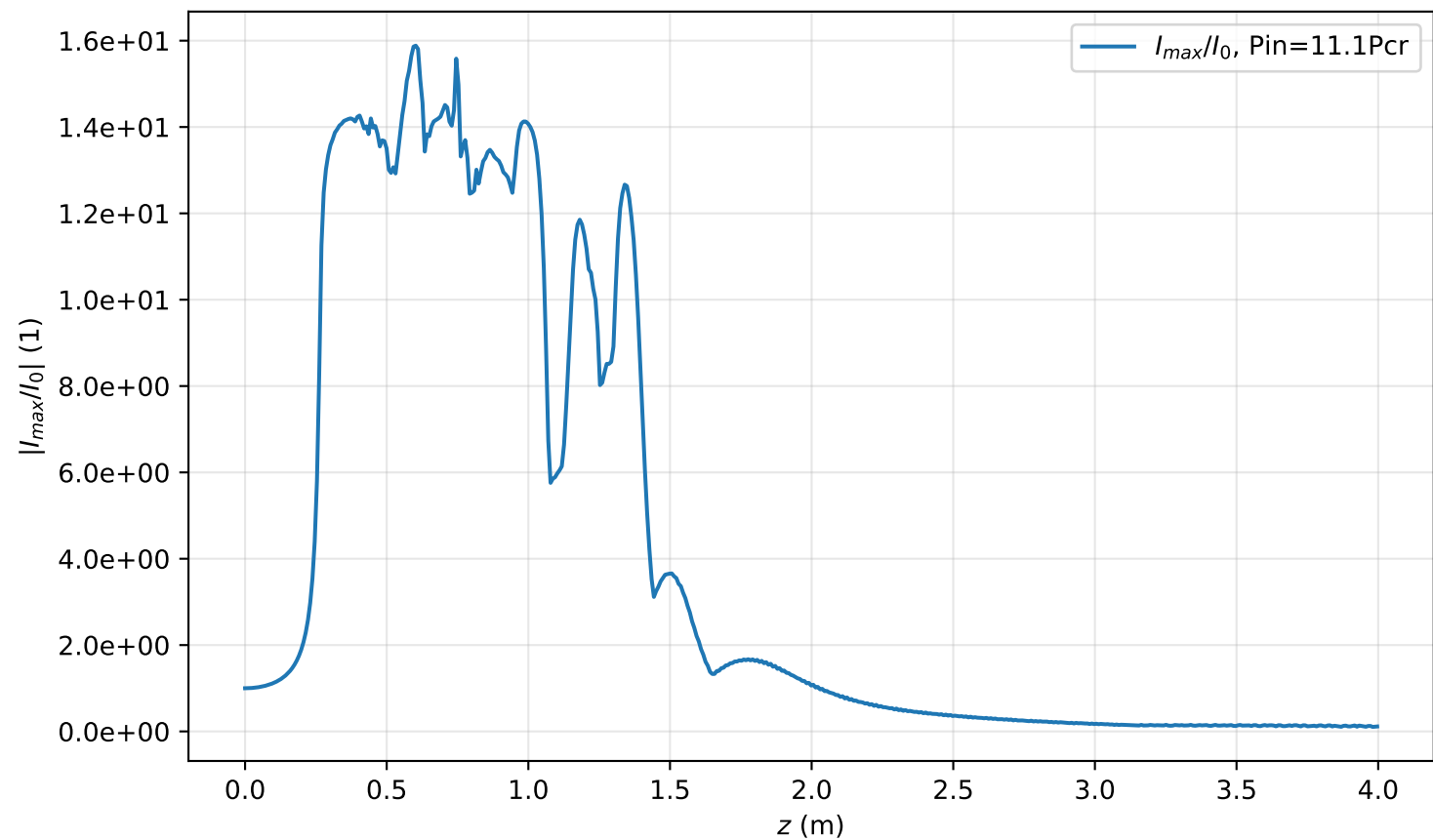
I_{max}(r=0, z)/I_0 , Pin=11.1Pcr
