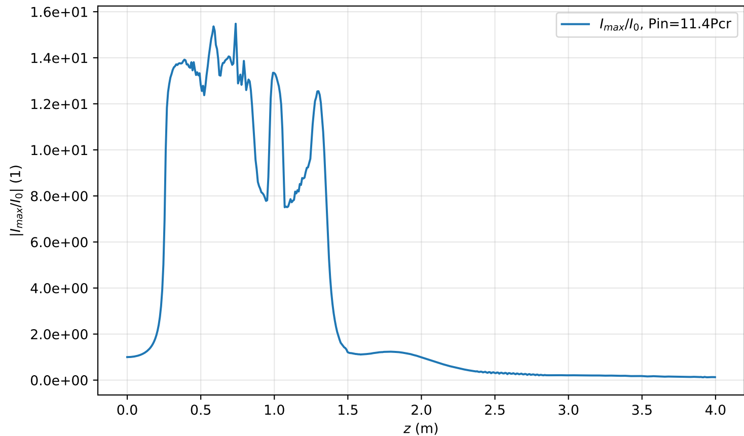
I_{max}(r=0, z)/I_0 , Pin=11.4Pcr
