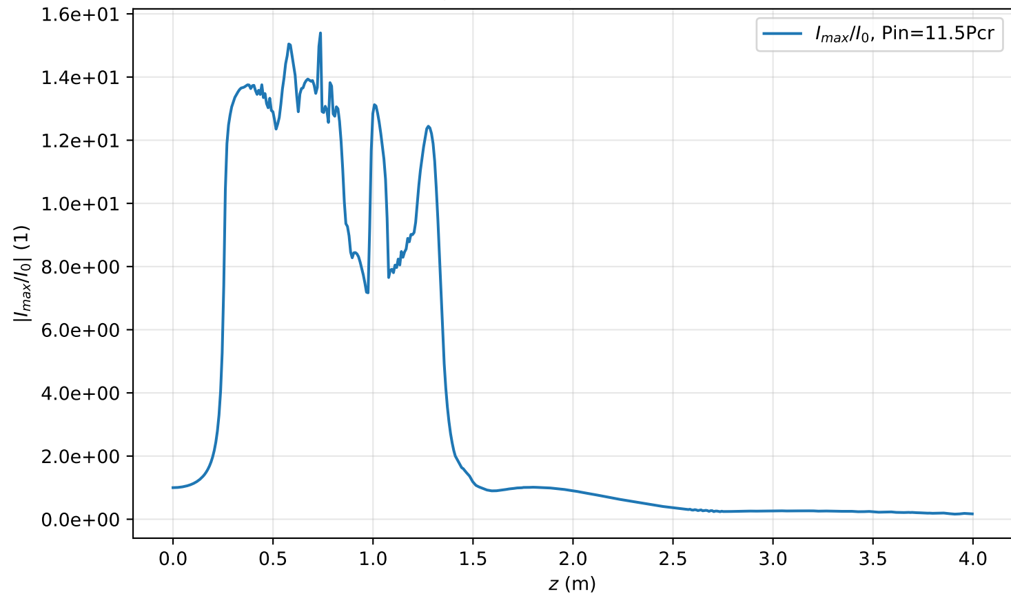
I_{max}(r=0, z)/I_0 , Pin=11.5Pcr
