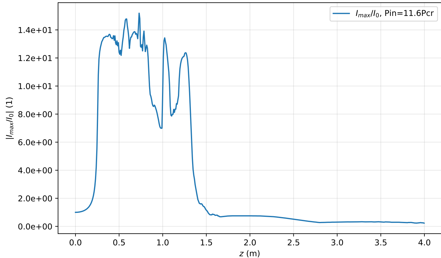
I_{max}(r=0, z)/I_0 , Pin=11.6Pcr
