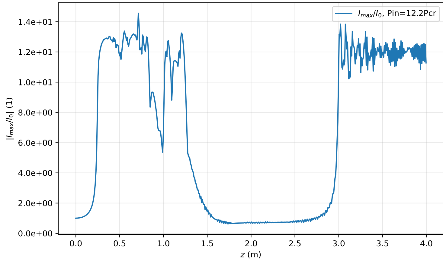
I_{max}(r=0, z)/I_0 , Pin=12.2Pcr
