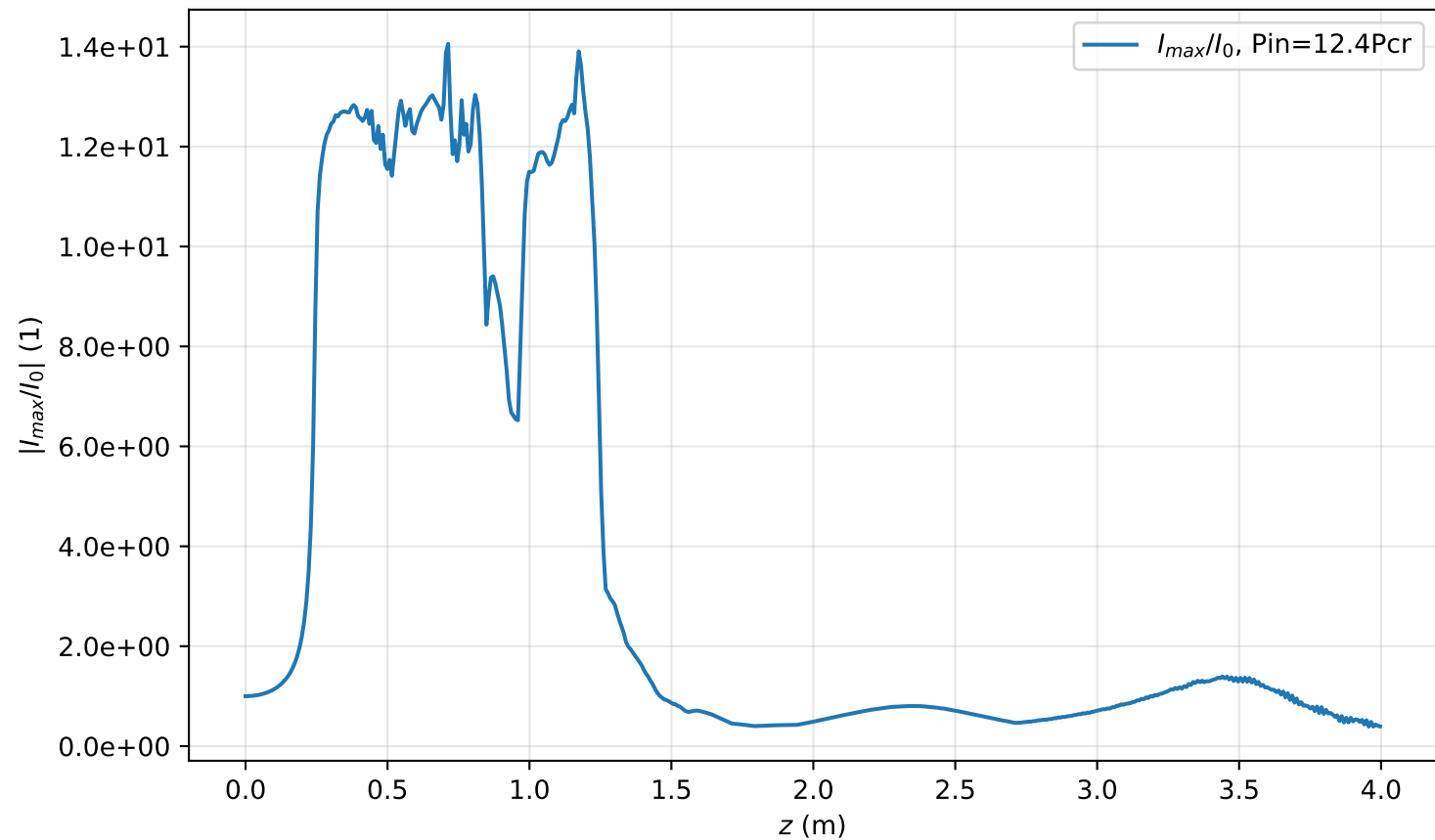
I_{max}(r=0, z)/I_0 , Pin=12.4Pcr
