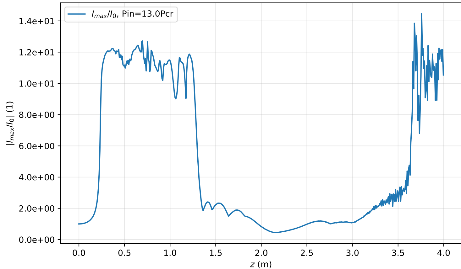
I_{\max}(r=0, z)/I_0 , Pin=13.0Pcr
