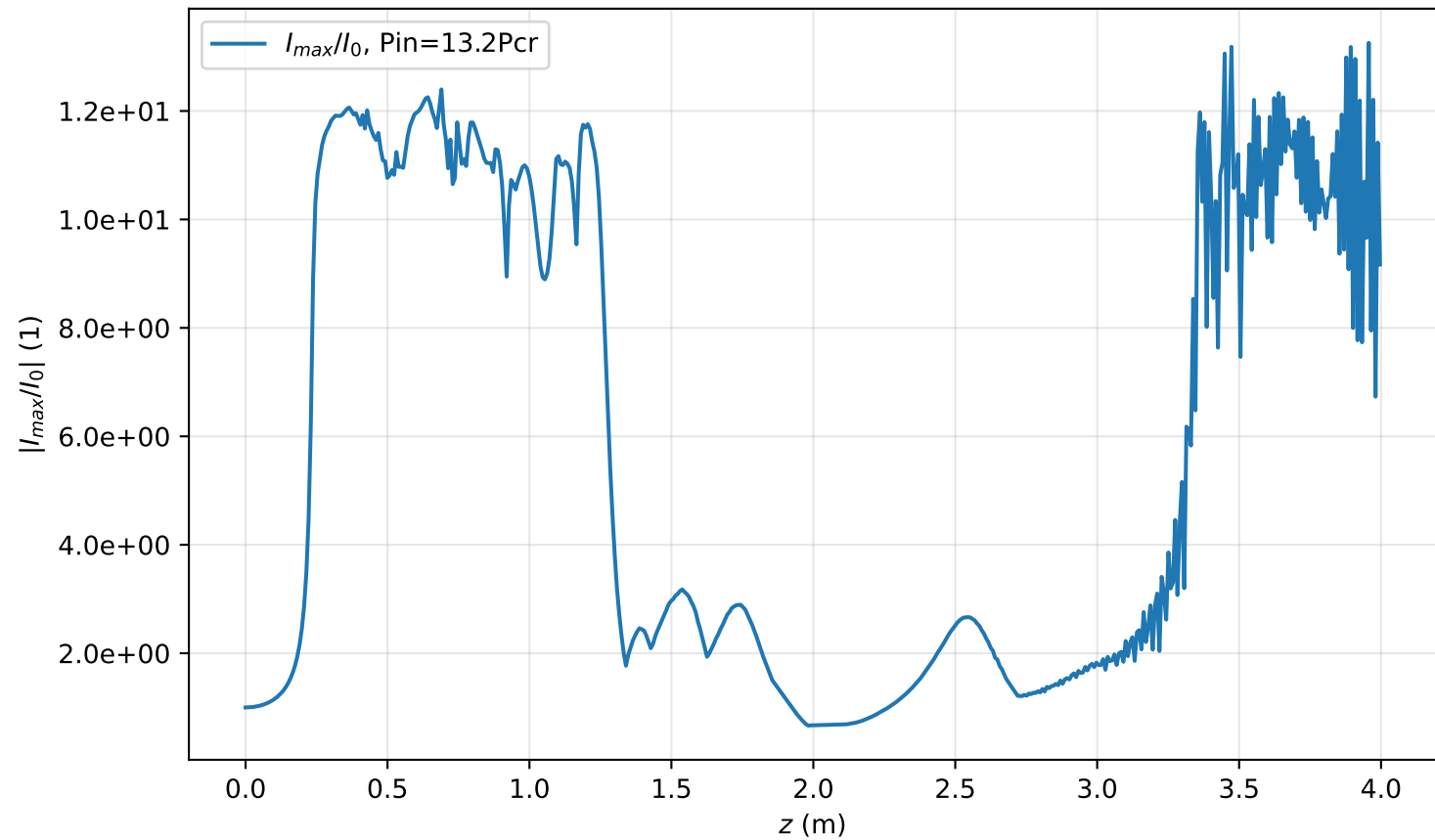
I_{\max}(r=0, z)/I_0 , Pin=13.2Pcr
