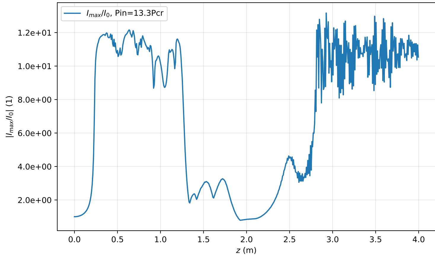
I_{\max}(r=0, z)/I_0 , Pin=13.3Pcr
