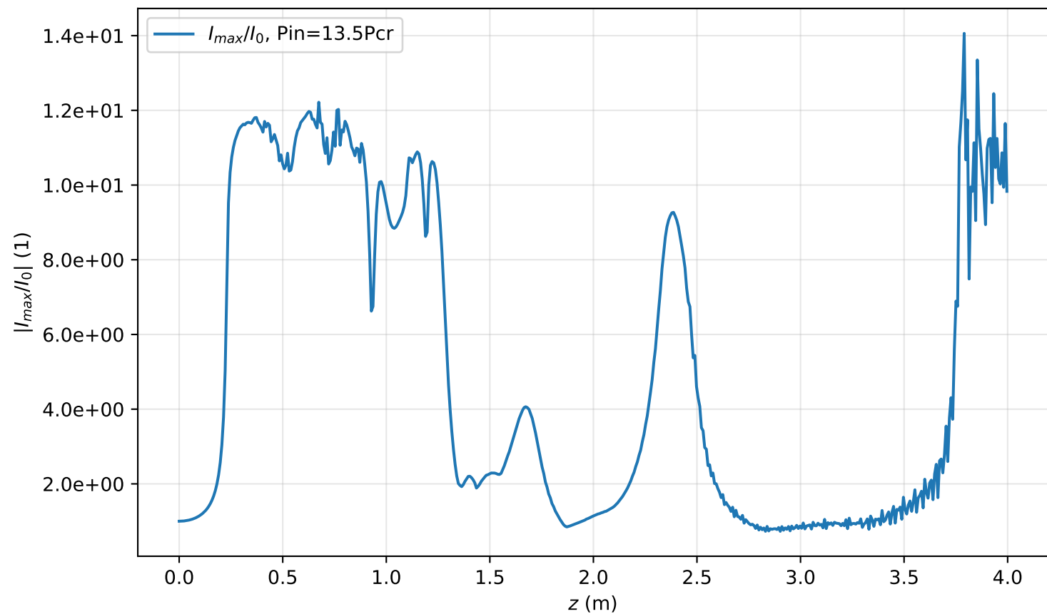
I_{max}(r = 0, z)/I_0 , Pin=13.5Pcr
