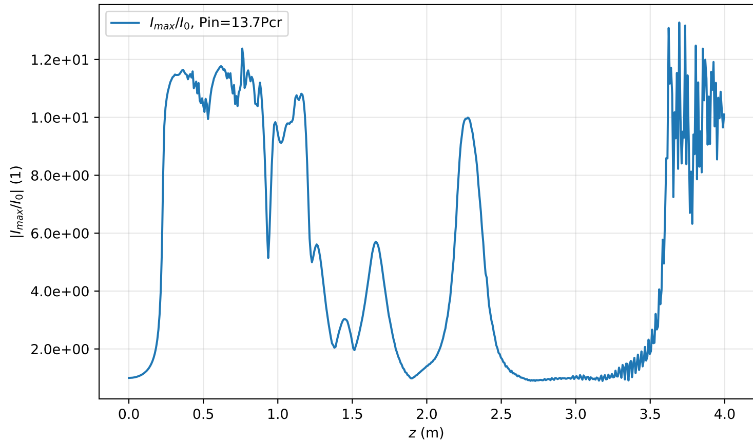
I_{\max}(r=0, z)/I_0 , Pin=13.7Pcr
