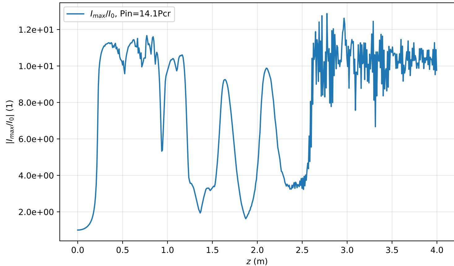
I_{max}(r=0, z)/I_0 , Pin=14.1Pcr
