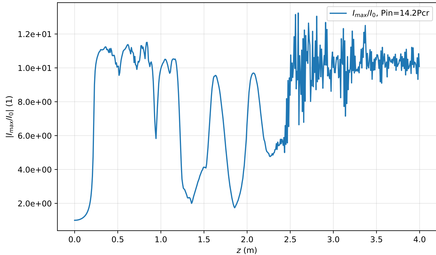
I_{\max}(r=0, z)/I_0 , Pin=14.2Pcr
