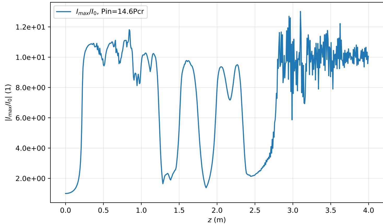
I_{\max}(r=0, z)/I_0 , Pin=14.6Pcr
