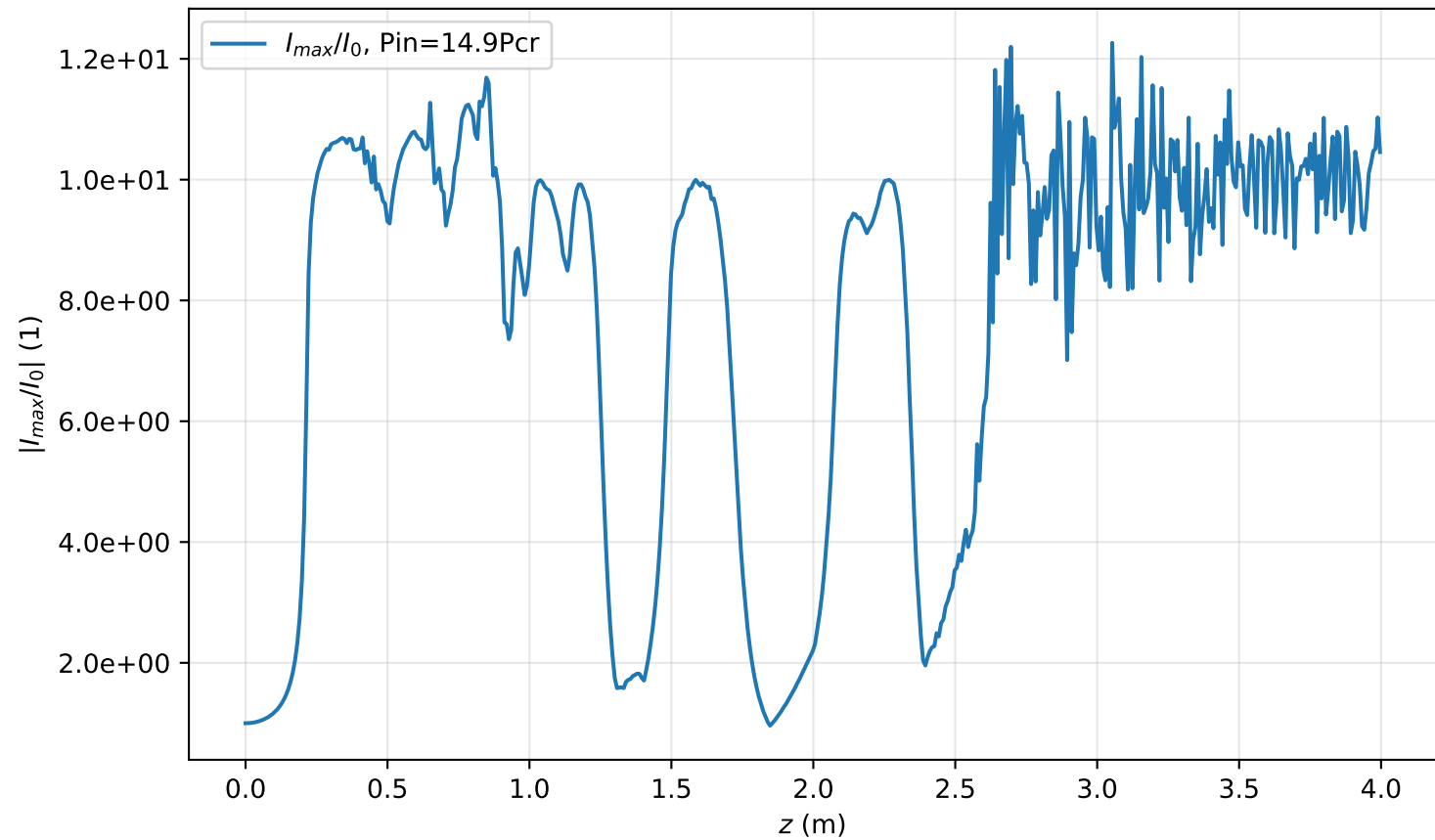
I_{\max}(r = 0, z)/I_0 , Pin=14.9Pcr
