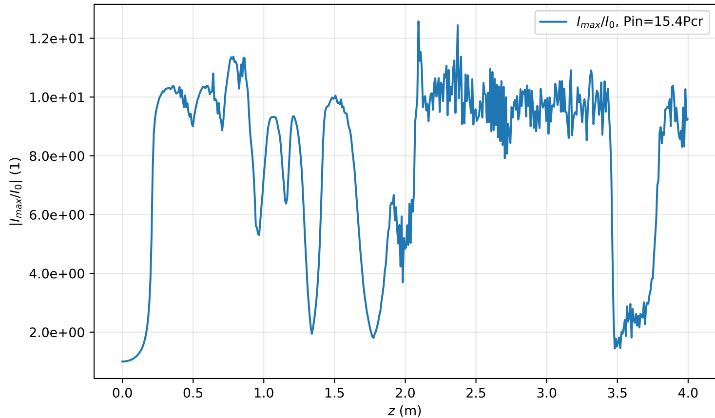
I_{max}(r=0, z)/I_0 , Pin=15.4Pcr
