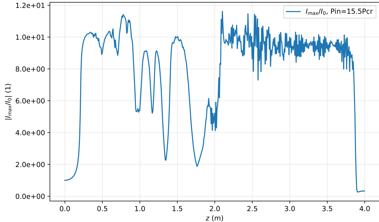
I_{max}(r=0, z)/I_0 , Pin=15.5Pcr
