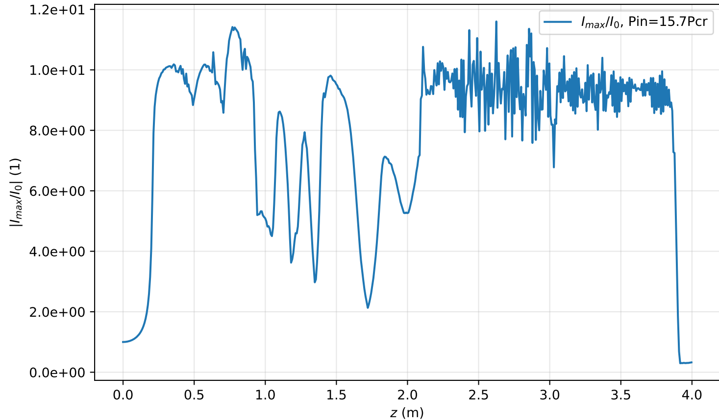
I_{\max}(r=0, z)/I_0 , Pin=15.7Pcr
