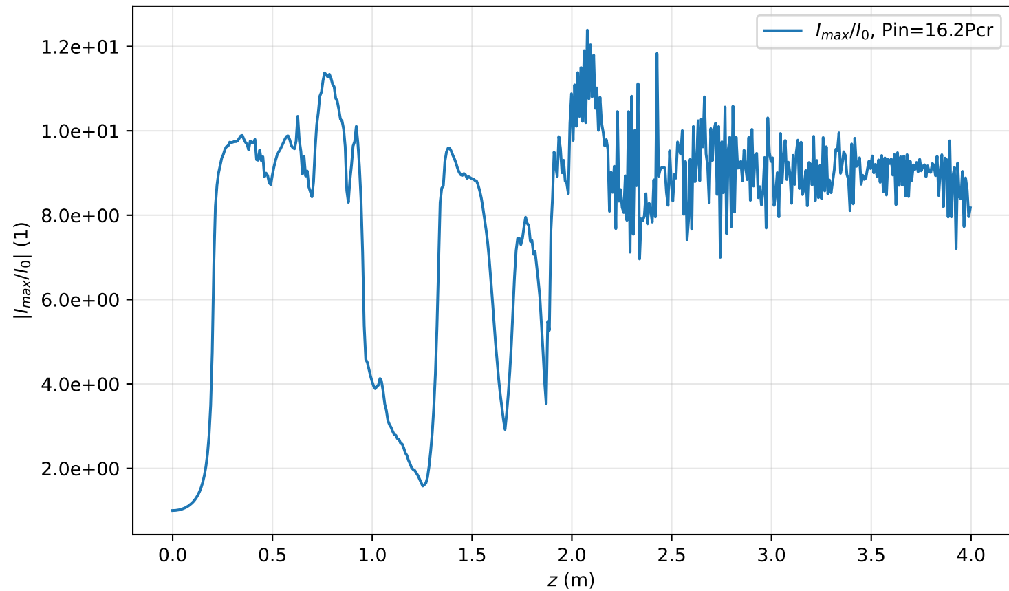
I_{\max}(r=0, z)/I_0 , Pin=16.2Pcr
