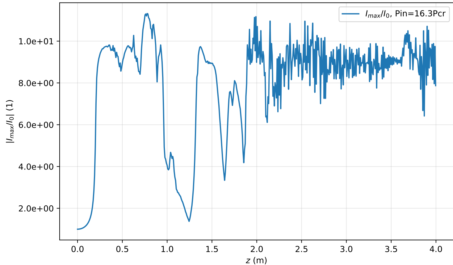
I_{\max}(r=0, z)/I_0 , Pin=16.3Pcr
