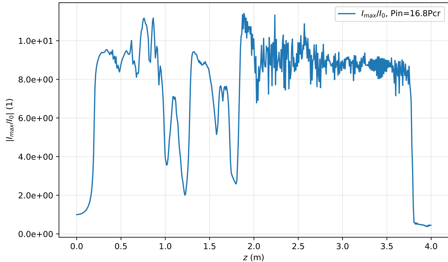
I_{max}(r=0, z)/I_0 , Pin=16.8Pcr
