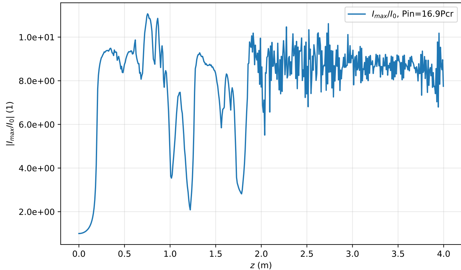
I_{max}(r=0, z)/I_0 , Pin=16.9Pcr
