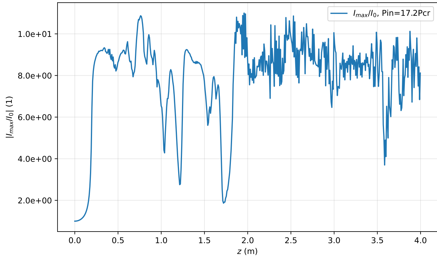
I_{max}(r=0, z)/I_0 , Pin=17.2Pcr
