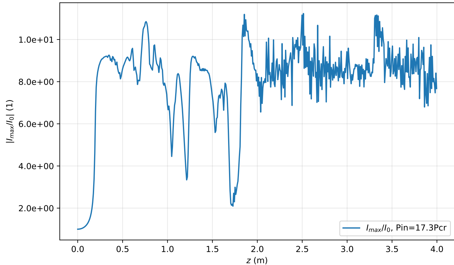
I_{max}(r=0, z)/I_0 , Pin=17.3Pcr
