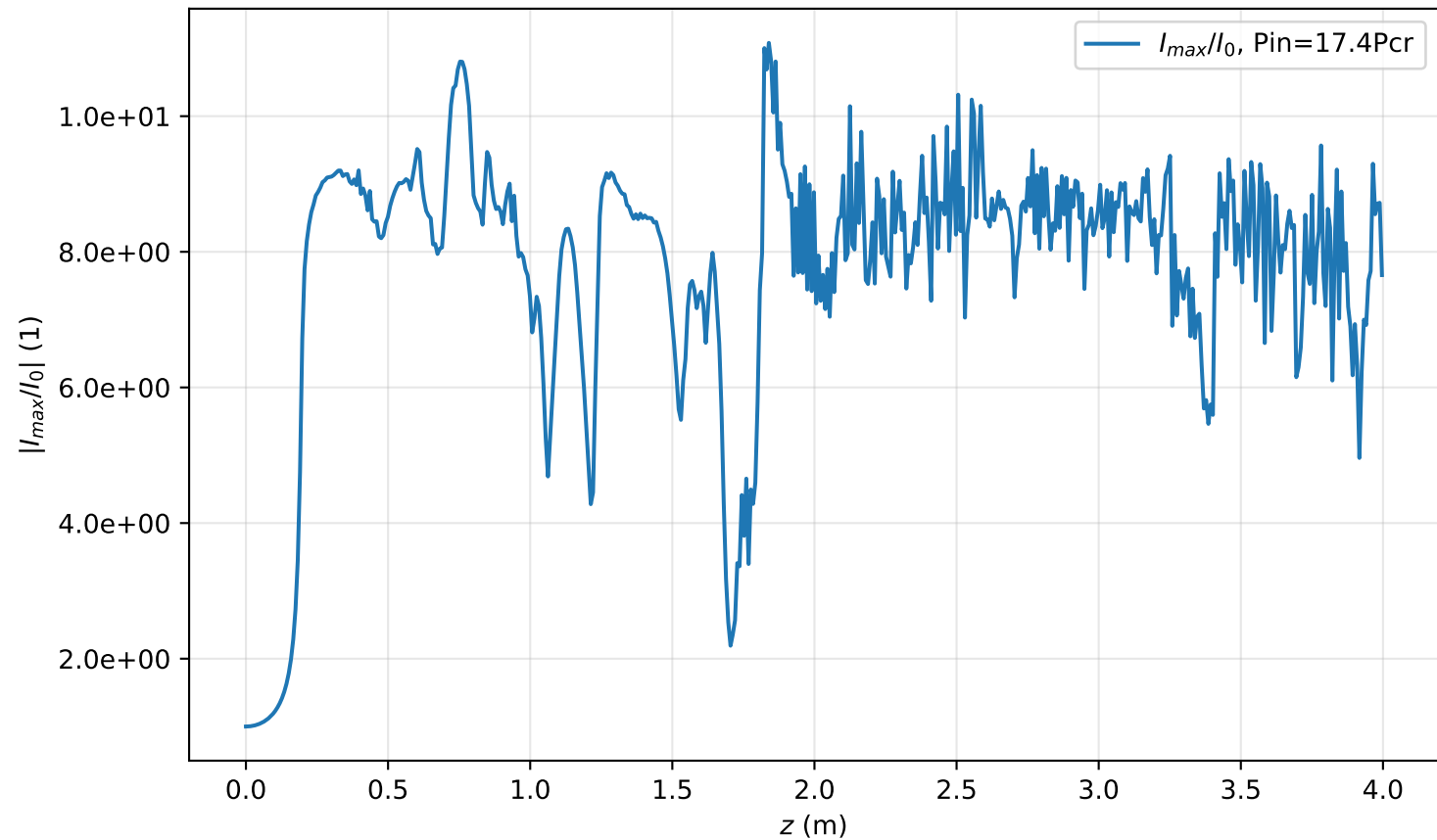
I_{max}(r=0, z)/I_0 , Pin=17.4Pcr
