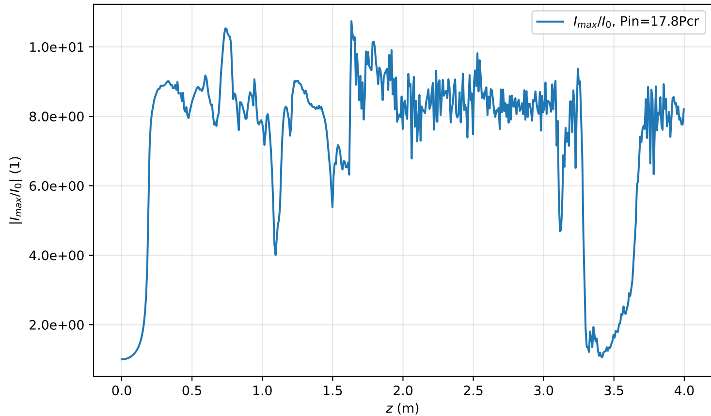
I_{\max}(r=0, z)/I_0 , Pin=17.8Pcr
