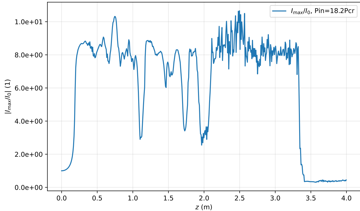
I_{max}(r=0, z)/I_0 , Pin=18.2Pcr
