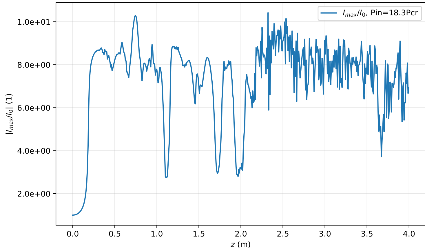
I_{max}(r=0, z)/I_0 , Pin=18.3Pcr
