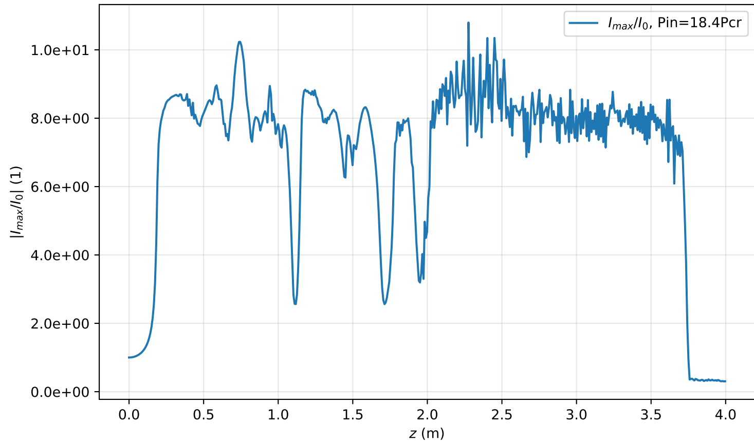
I_{max}(r=0, z)/I_0 , Pin=18.4Pcr
