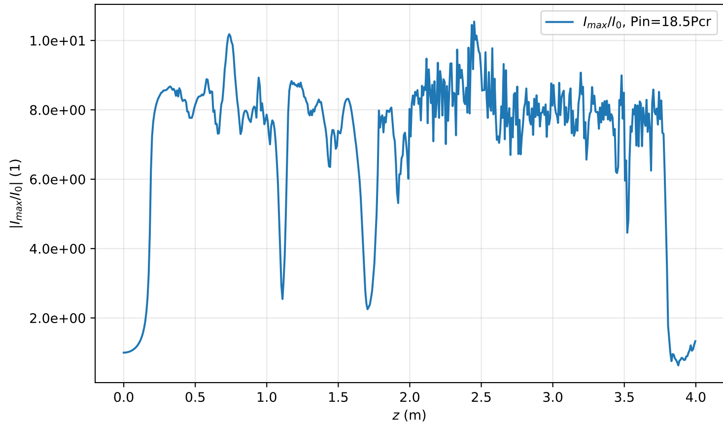
I_{max}(r=0, z)/I_0 , Pin=18.5Pcr
