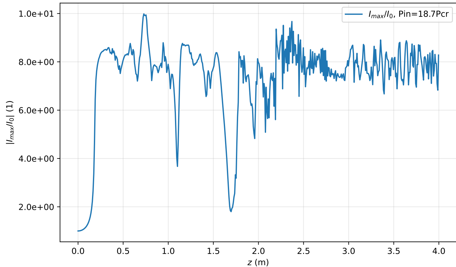
I_{max}(r=0, z)/I_0 , Pin=18.7Pcr
